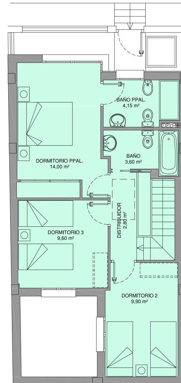
PLANTA ALTA
