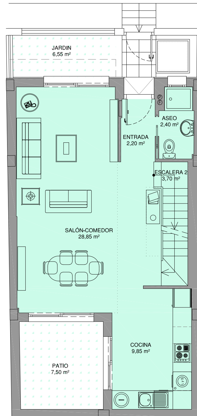
PLANTA BAJA
